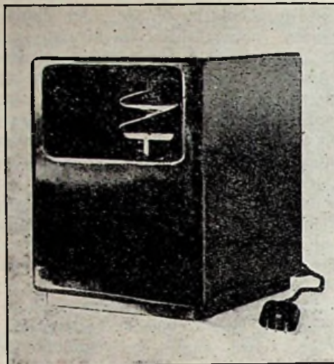
Fig. 4. Nieuwste televisietoestel van Te-Ka-De (Telehor). Men ziet het beeld, als men op de spiegelschroef kijkt. Zie over de spiegelschroef R.E. 1930 No. 42.
