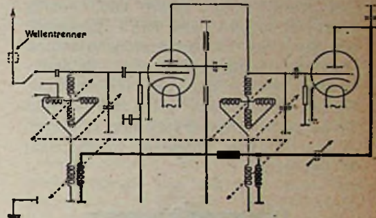
Fig. 1. Schakelschema van den 3-lamps-kwaliteitsontvanger „Siemens 35” met dubbele terugkoppeling, welke automatisch gelijktijdig met de afstemming wordt ingesteld en verder met een condensator met de hand regelbaar is. Het genereren der hoogfrequentlamp is door het aanbrengen van een weerstand onderdrukt. Het toestel heeft een ingebouwd zeeffkring, welke overgeschakeld kan worden als afgestemde antennekring. Verder is een toonzeeff ingebouwd, welke tusschen 4000 en 5000 Hertz afsijdt.
